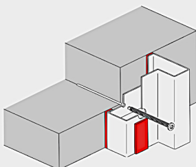
Detalle instalación
